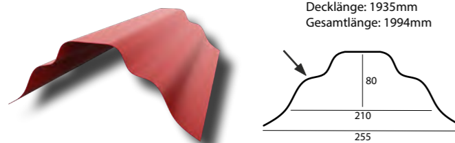
7. Einfacher First - Flachfirst 200 TYP 2
