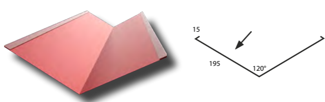
19. Seitliches Ortgangblech
