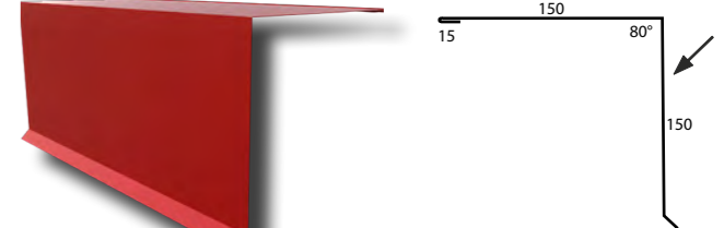
24. Pultdachfirst 150/150
