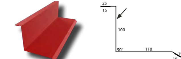
12. Wandanschluss / Maueranschluss TYP 3
