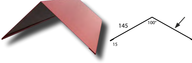
8. Flachfirst TYP 3
