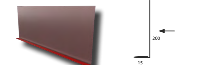
23. Unteres Traufblech / Rinneneinlaufblech
