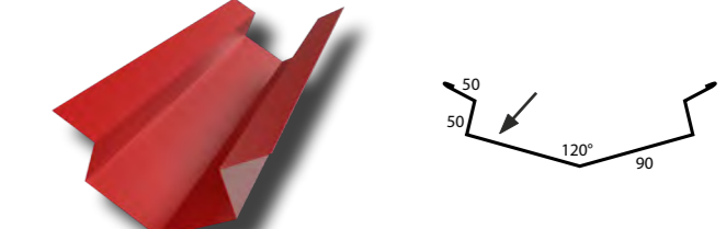
20. Kaminleiste / - Anschluss
