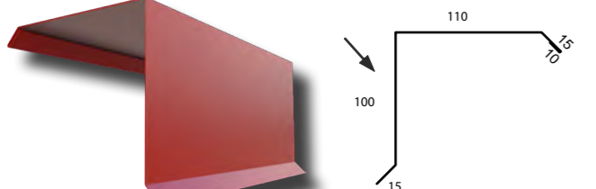
13. Ortgangblech
