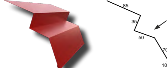
10 IRYD Startleiste
