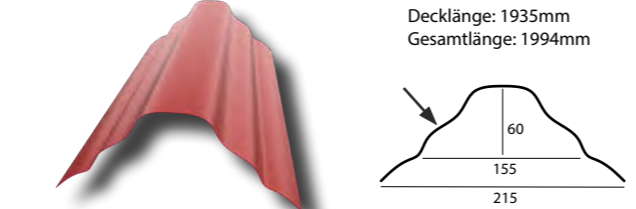
6. Einfacher First - Flachfirst TYP 1
