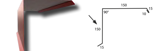
18. Kehlrinne (tief)
