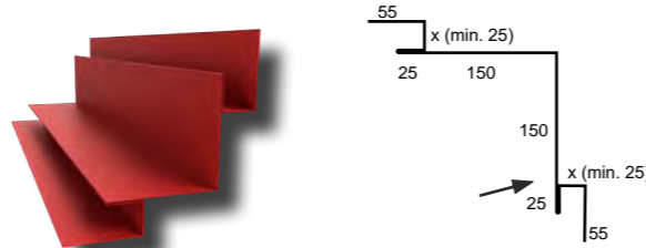
8. Tropfleiste
