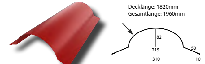
5. Omega - Rundfirst groß
